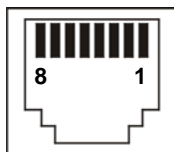
Port RJ45 du contrôleur vue de face
