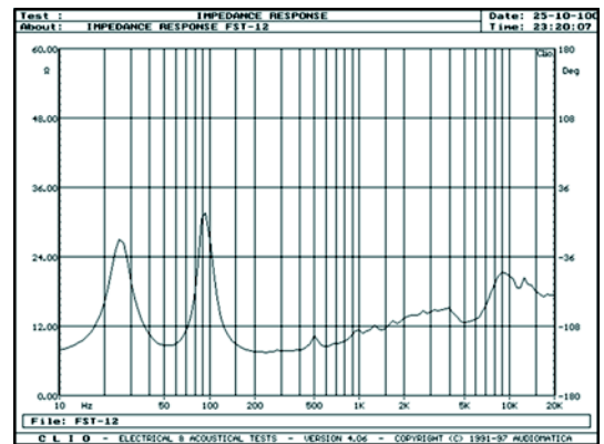
Courbe d'Impédance
